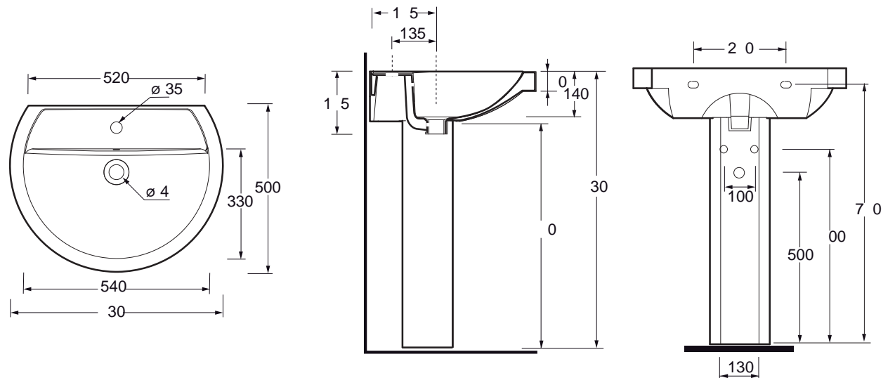
Art. SPL1 Lavabo Washbasin
